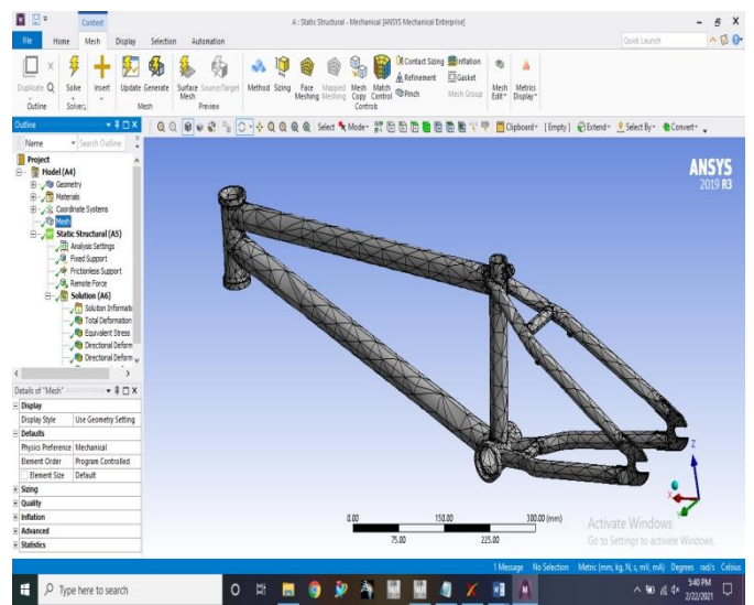
FIG12-MESH
